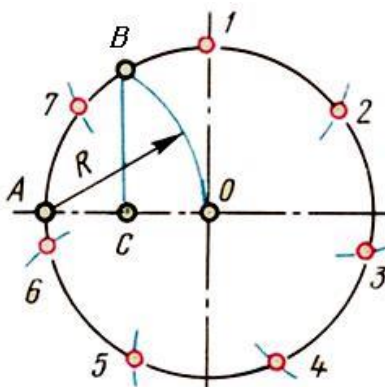
Рис. 9. Деление окружности на 7 равных частей
