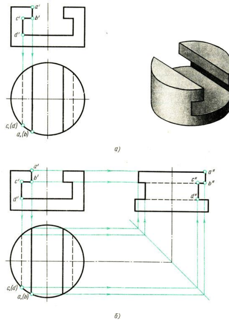
Рис. 1. Построение проекций выреза на цилиндре
