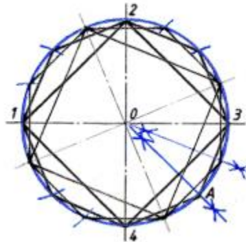
Рис.3. Деление окружности на 16 равных частей.
