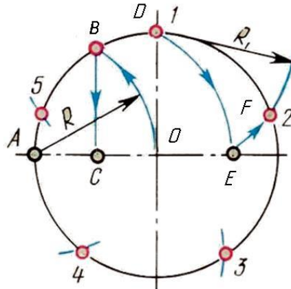
Рис. 7. Деление окружности на 5 равных частей
