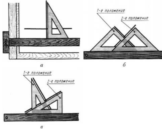
Рис. 2.2. Построение прямых углов с помощью угольника
