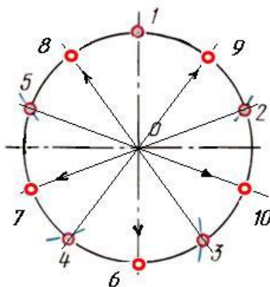
Рис. 8. Деление окружности на 10 равных частей
